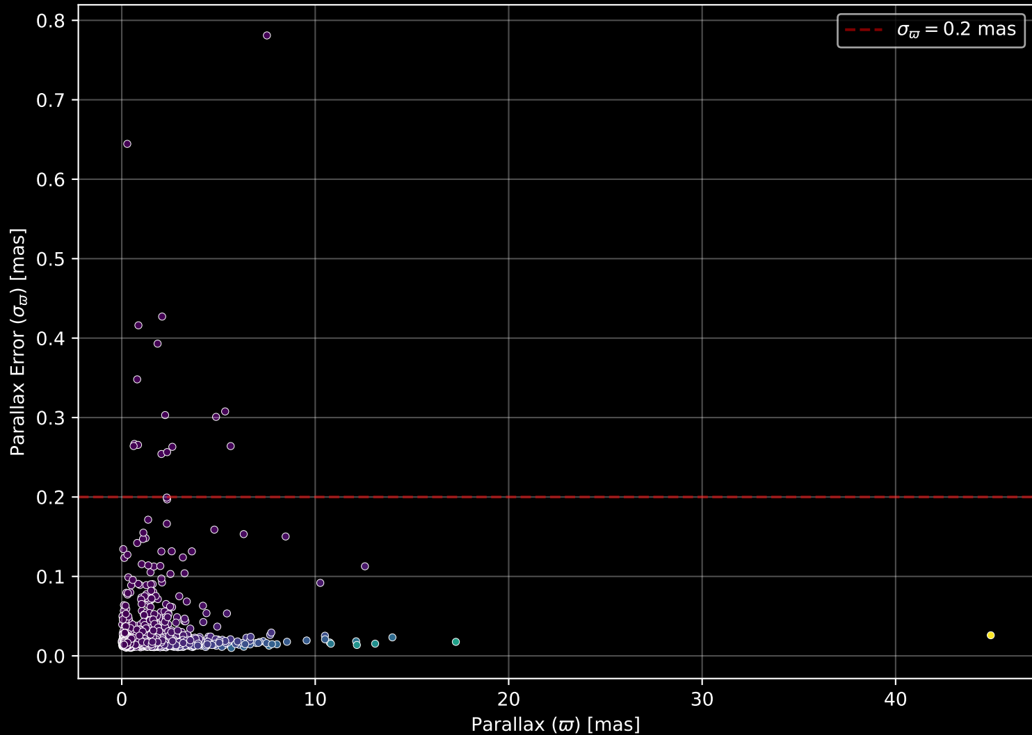
GALAH DR4 Field: [-11] Parallax Quality (n= 3166)
