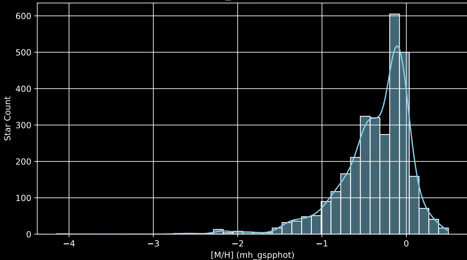
GALAH DR4 Field: [-11] [M/H] (mh_gspphot) (n= 3126)
