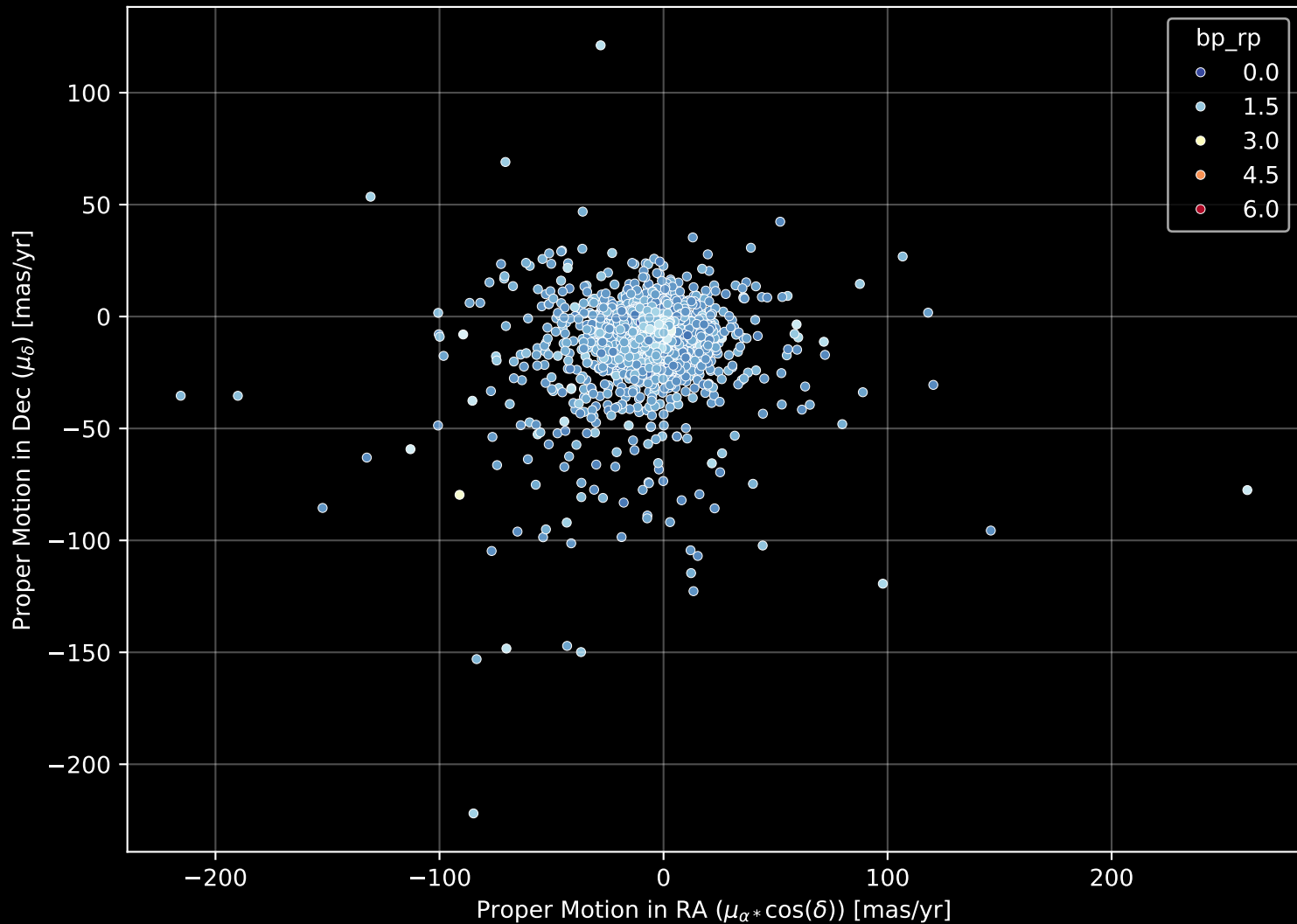
GALAH DR4 Field: [-11] Proper Motion Diagram (n= 3166)
