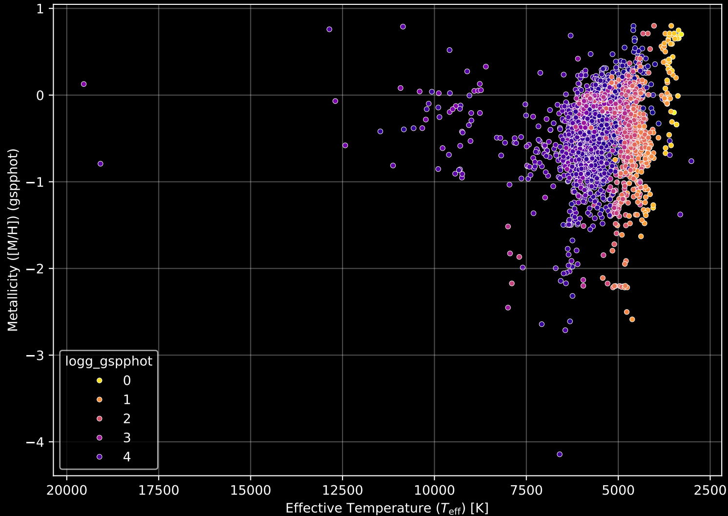
GALAH DR4 Field: [-11] Stellar Population Parameters (n= 3166)
